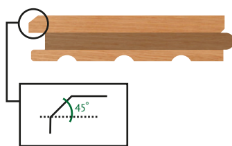
T&G 4s MB4 (Microbiselado)
